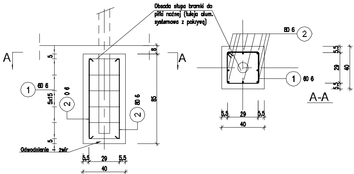
Zestawienie stali dla fundamentu/1szt
