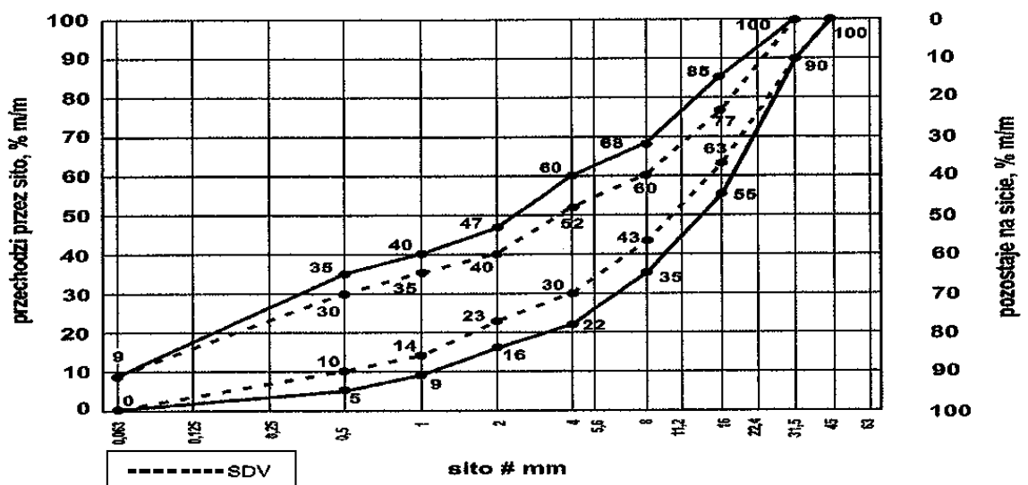
Rys. 5.9.1. Krzywe graniczne uziarnienia mieszanki kruszywa niezwiązanego 0/31,5 mm do warstw podbudowy zasadniczej
