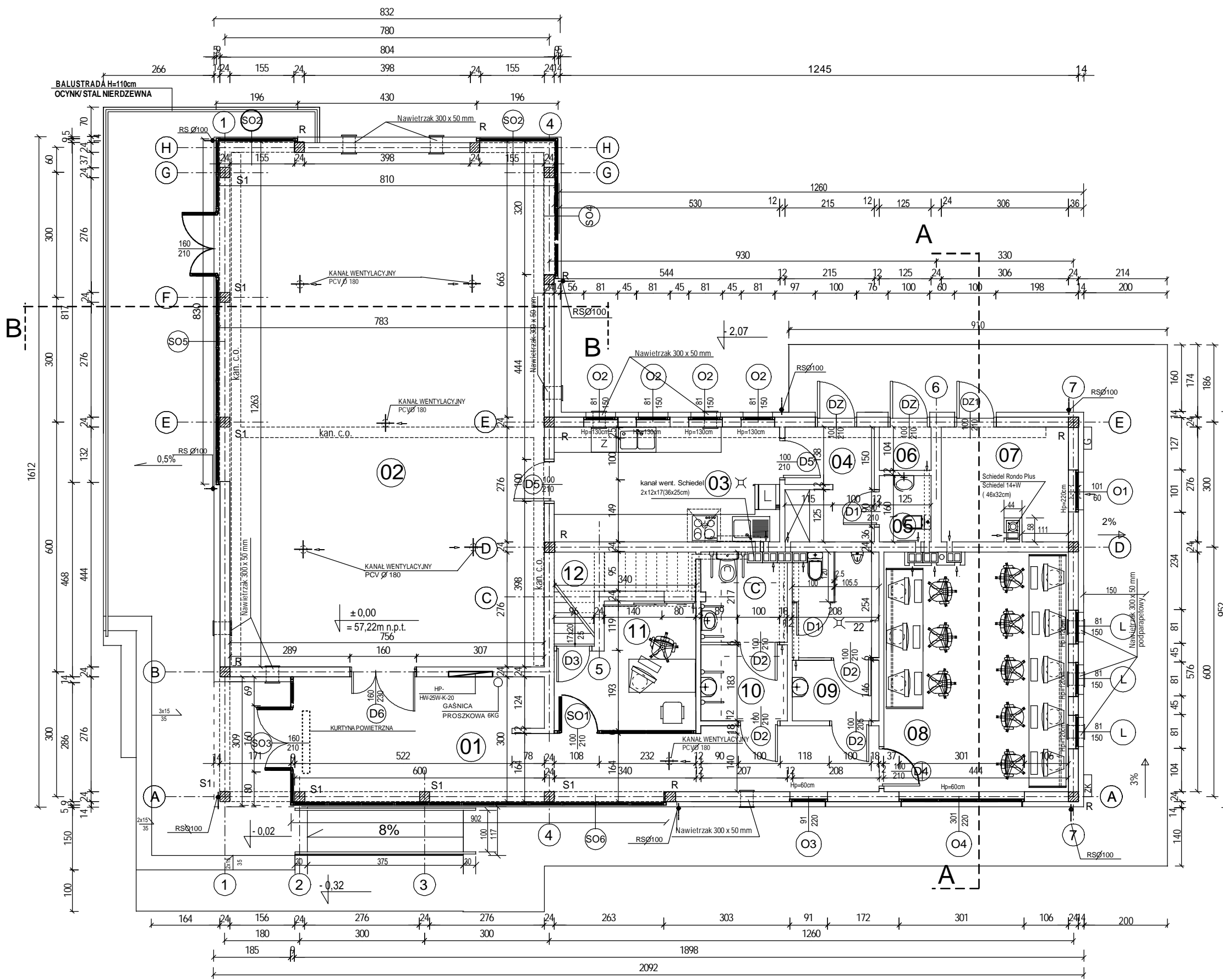
RZUT PRZYZIEMIA 1:100
