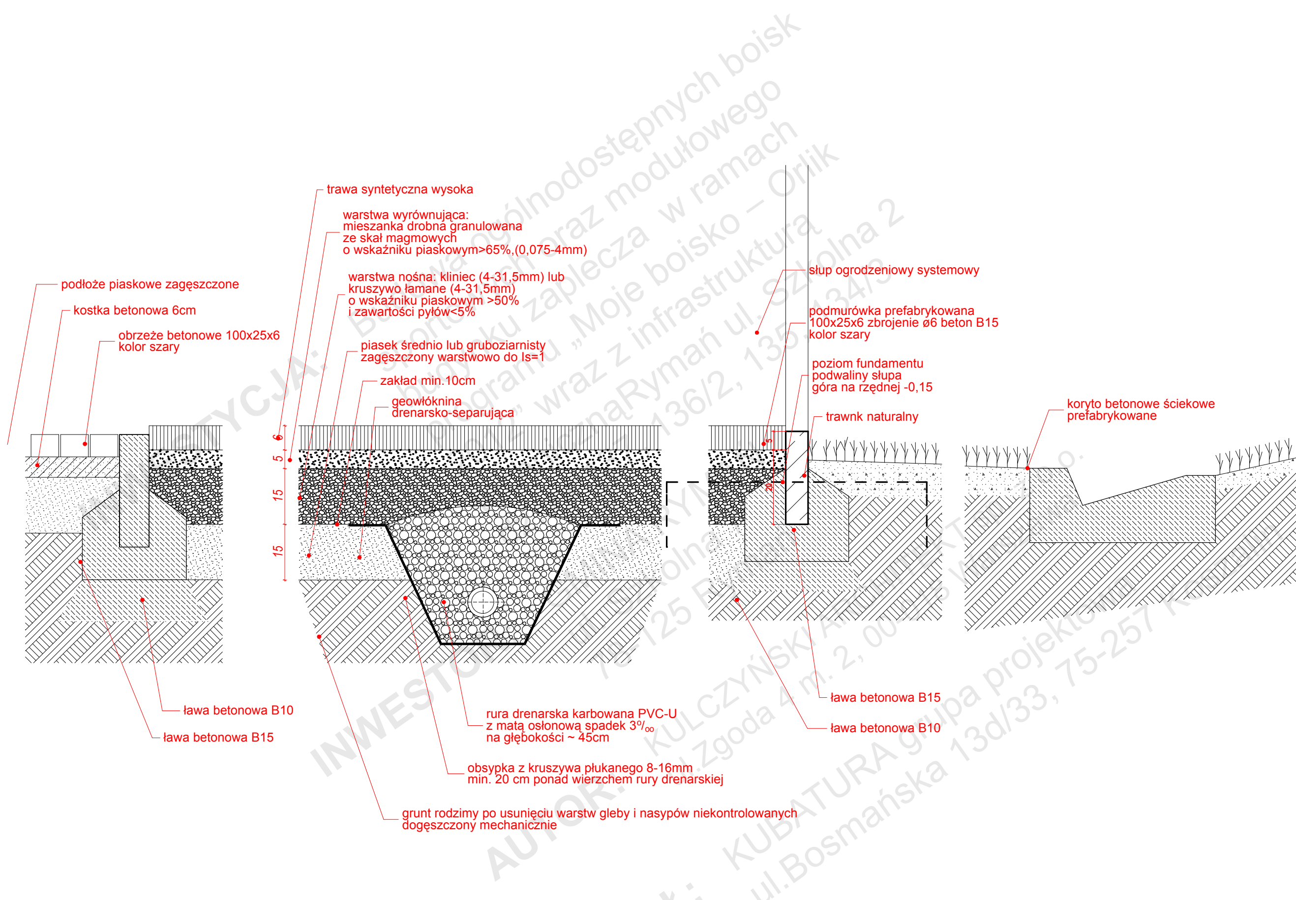
POŁĄCZENIE Z NAWIERZCHNIĄ Z KOSTKI BETONOWEJ
