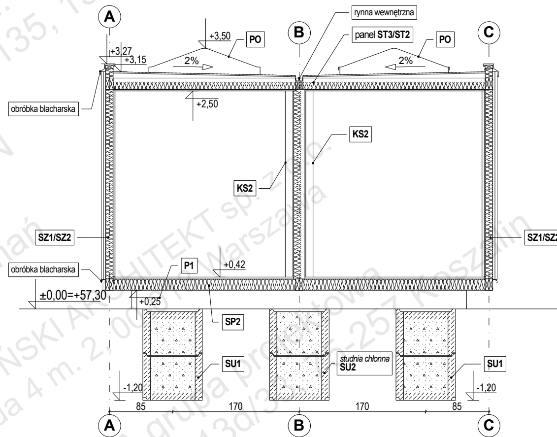
PRZEKRÓJ PIONOWY II-II
