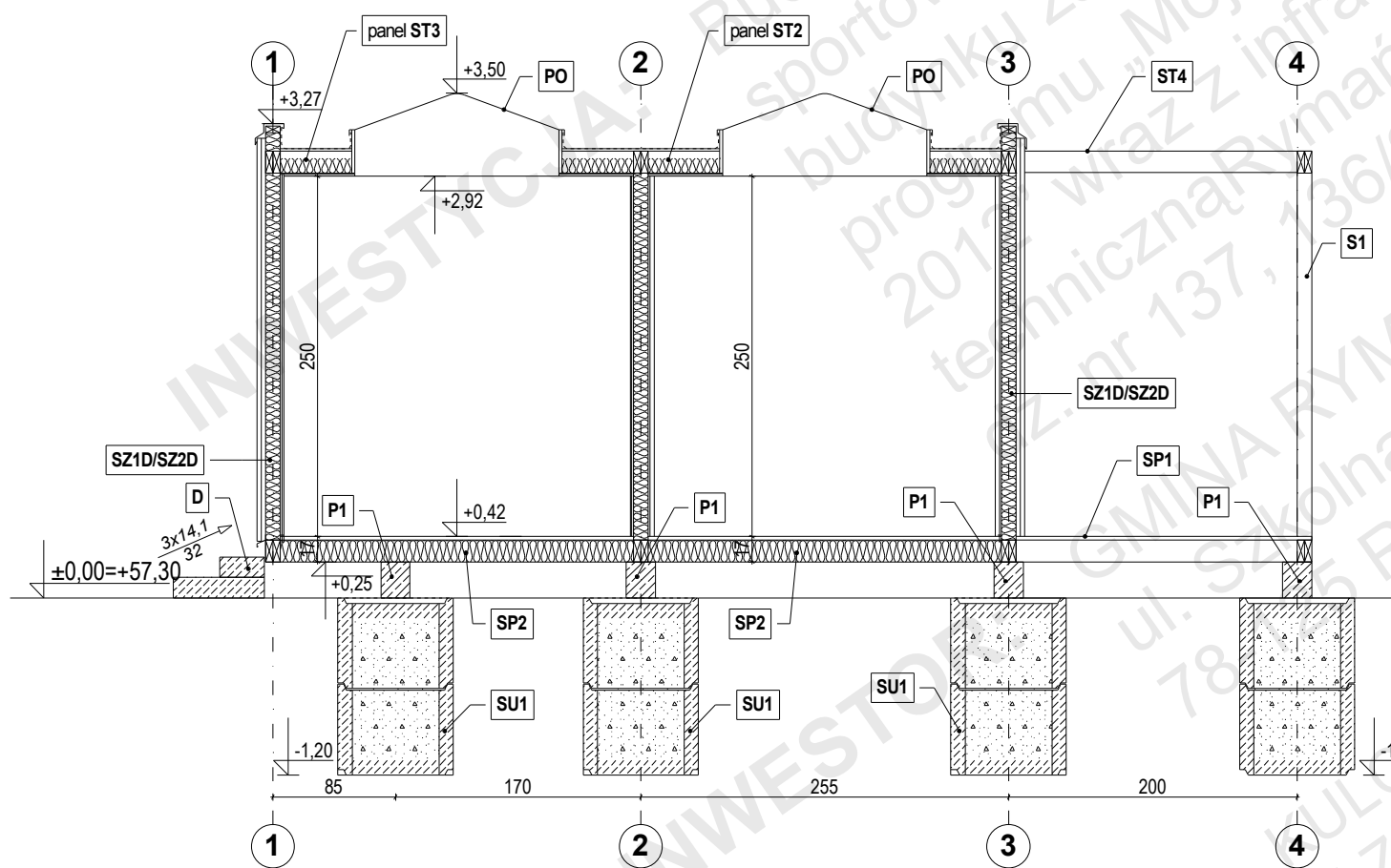
PRZEKRÓJ PIONOWY I-I
